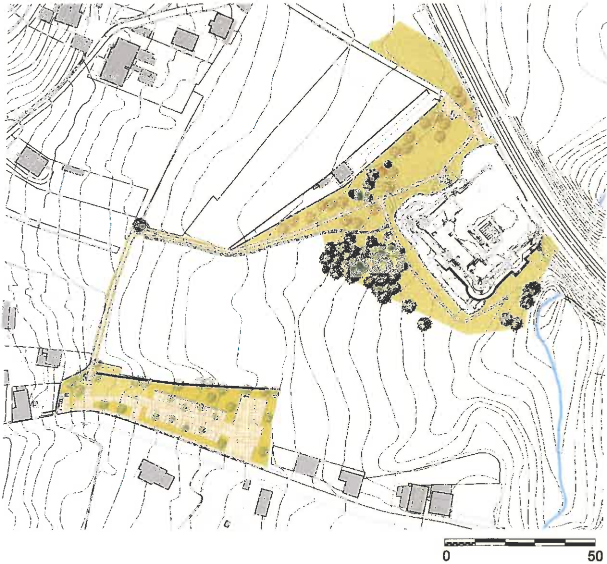
Vista xeral do proxecto de acondicionamento exterior do castelo de A Rocha Forte (r v r, 2014)
