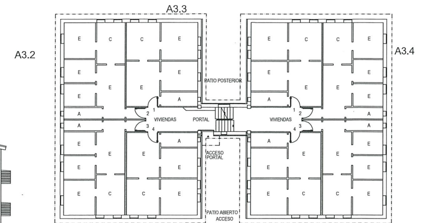
PLANTA BAIXA UNIDADE 1. ESTADO ACTUAL
