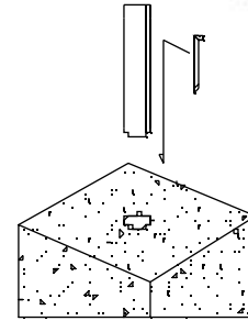
DETALLE ANCLAJE DE POSTE A ZAPATA DE HORMIGÓN CON GUÍA
