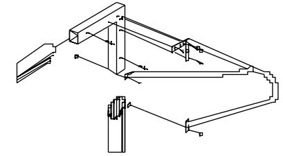
DETALLE UNIÓN POSTE-LARGUERO Y ARQUILLO RED.
