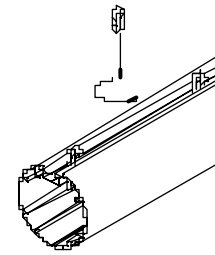
DETALLE ENGANCHE DE RED
