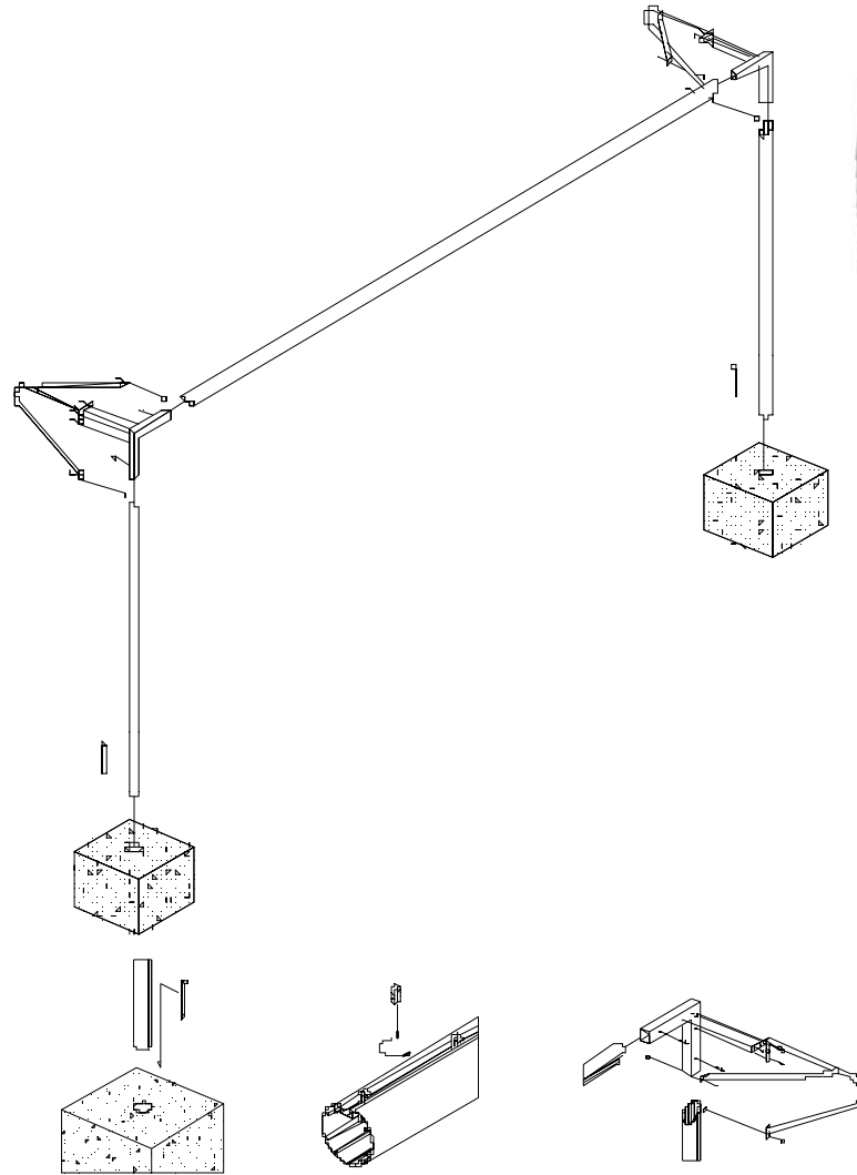
DETALLE ANCLAJE DE POSTE A ZAPATA DE HORMIGÓN CON GUSAS
